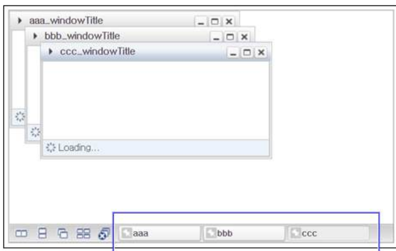
그림 40-32 고정된 윈도우가 없는 경우
