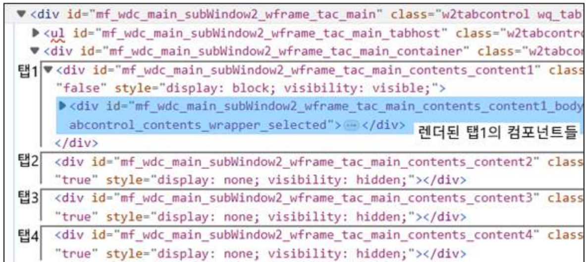
그림 37-7 초기 렌더링 결과
