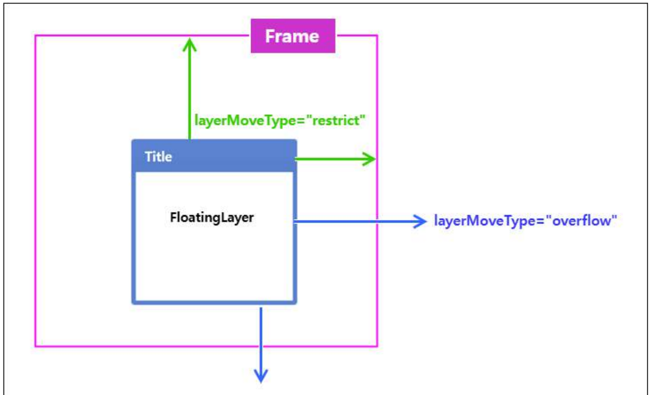
그림 30-5 layerMoveType 속성 설정에 따른 FloatingLayer의 이동 범위
