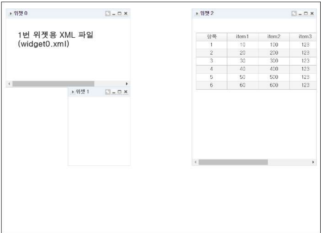
그림 39-24 WidgetContainer 생성 결과 (세 개의 위젯 포함)
