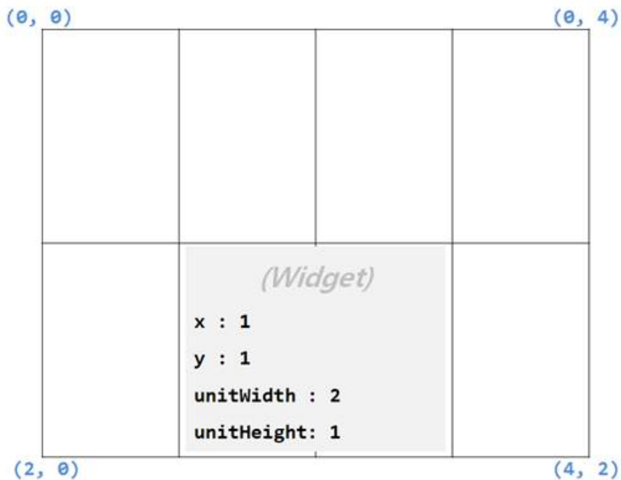
그림 39-2 좌표계 및 좌표계 상에 위젯 생성
