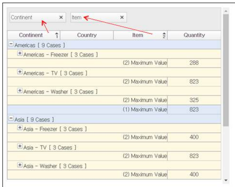
그림 26-179 헤더 드래깅을 통한 그룹핑
