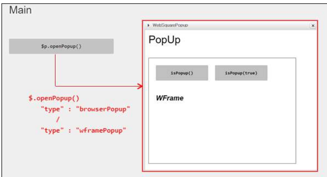
그림 53-16 팝업에 포함된 WFrame에서 자신 및 부모 화면이 팝업인지 여부를 확인
