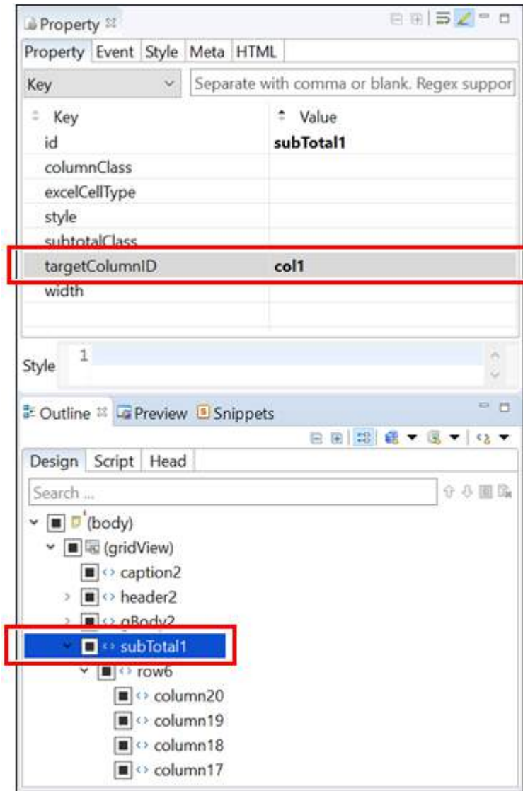
그림 26-5 subTotal의 targetColumnID 지정
