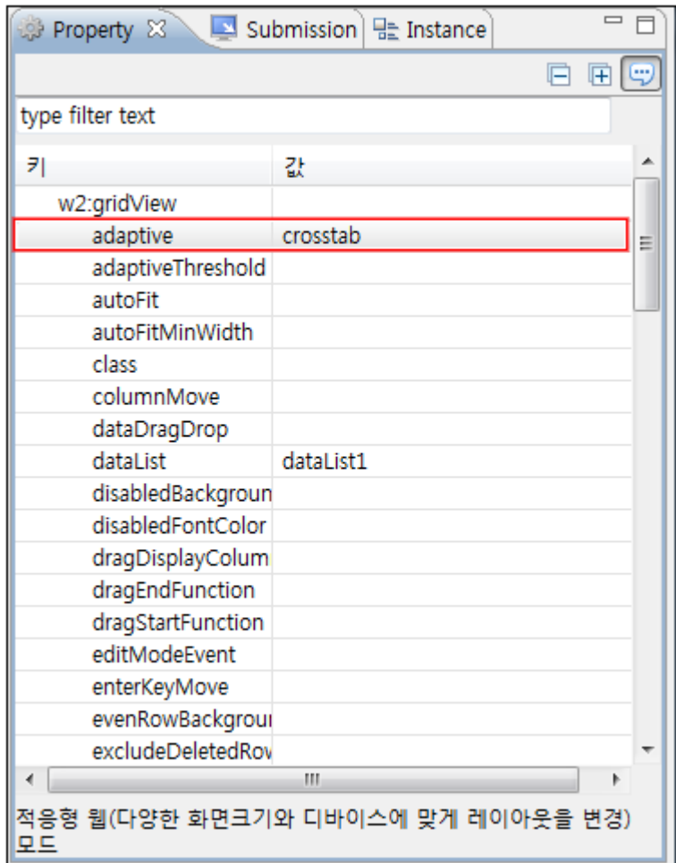
그림 57-6 GridView Property View
