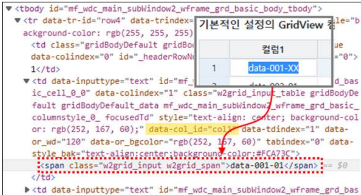
그림 27-9 &lt;tr&gt; 노드 확장
