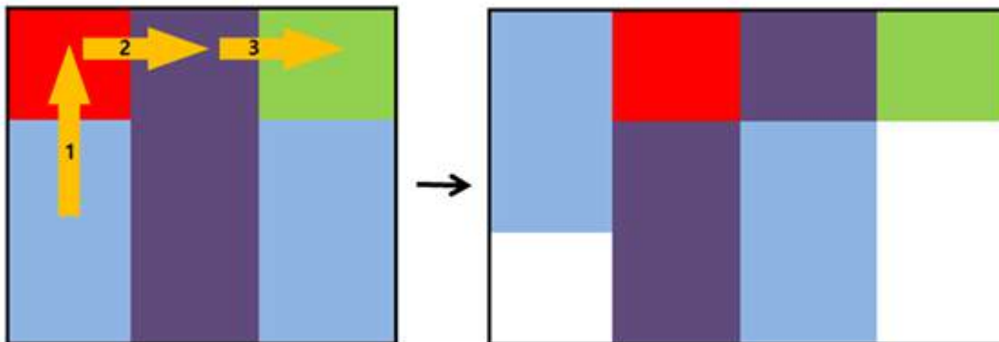
그림 39-8 rows 및 unitWidthPixel 속성으로 구성된 좌표계에서 위젯의 이동
