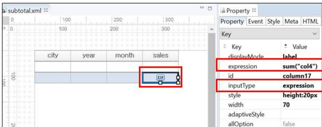
그림 26-6 subTotal을 표시할 컬럼의 inputType 및 expression 속성 지정
