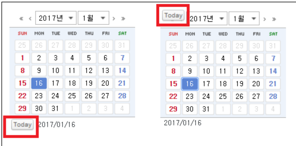
그림 3-3 topLayout="false" Vs. topLayout="true"
